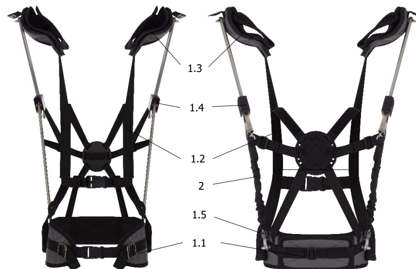
ВИД СПЕРЕДИ
